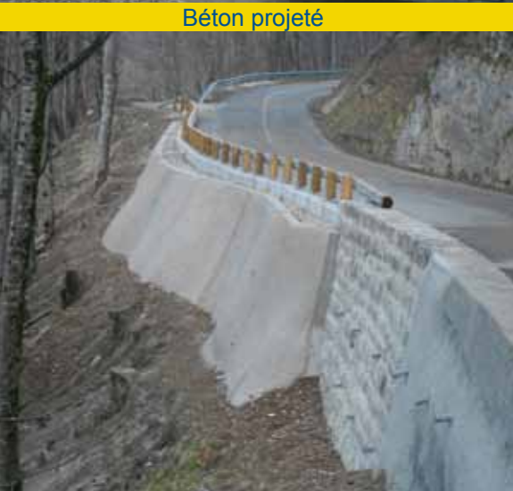
Paroi clouée
